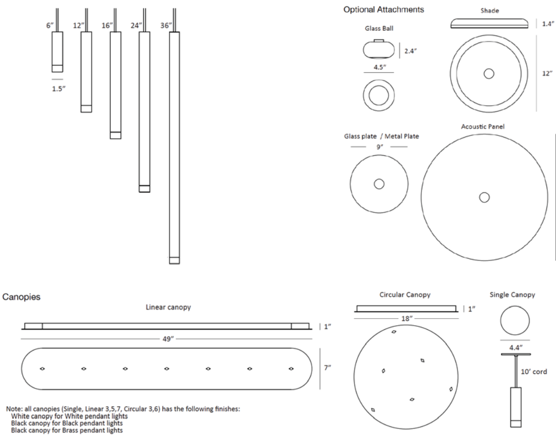
Combi Pendant Dimensions
